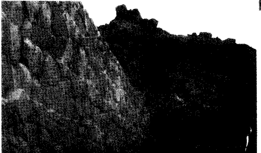
صورة رقم (٤٤) : يظهر فيها (السد الثالث) من سداد الحجاج بن يوسف أيضاً. وهو لا يختلف في هندسته عن السدين (الأول والثاني). ولا زال هذا السد بحالة جيدة. ولم يندم منه شيء. وطوله (٦٠) م وارتفاعه (٨.٥) م وعرضه من أعلاه (٤.١٥) م. أنظر الفاكهي (١٧٠/٤).
