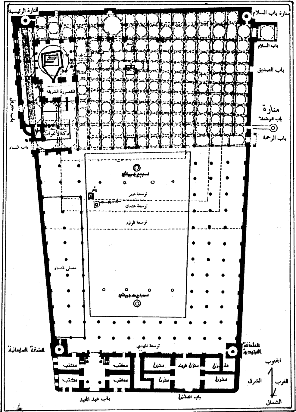
رسم توضيحي للمسجد بعد العمارة الجديدة . (٢)
